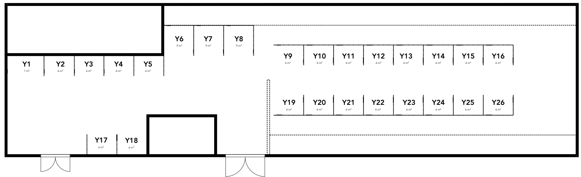
BOTTENPLAN, skala 1:225
